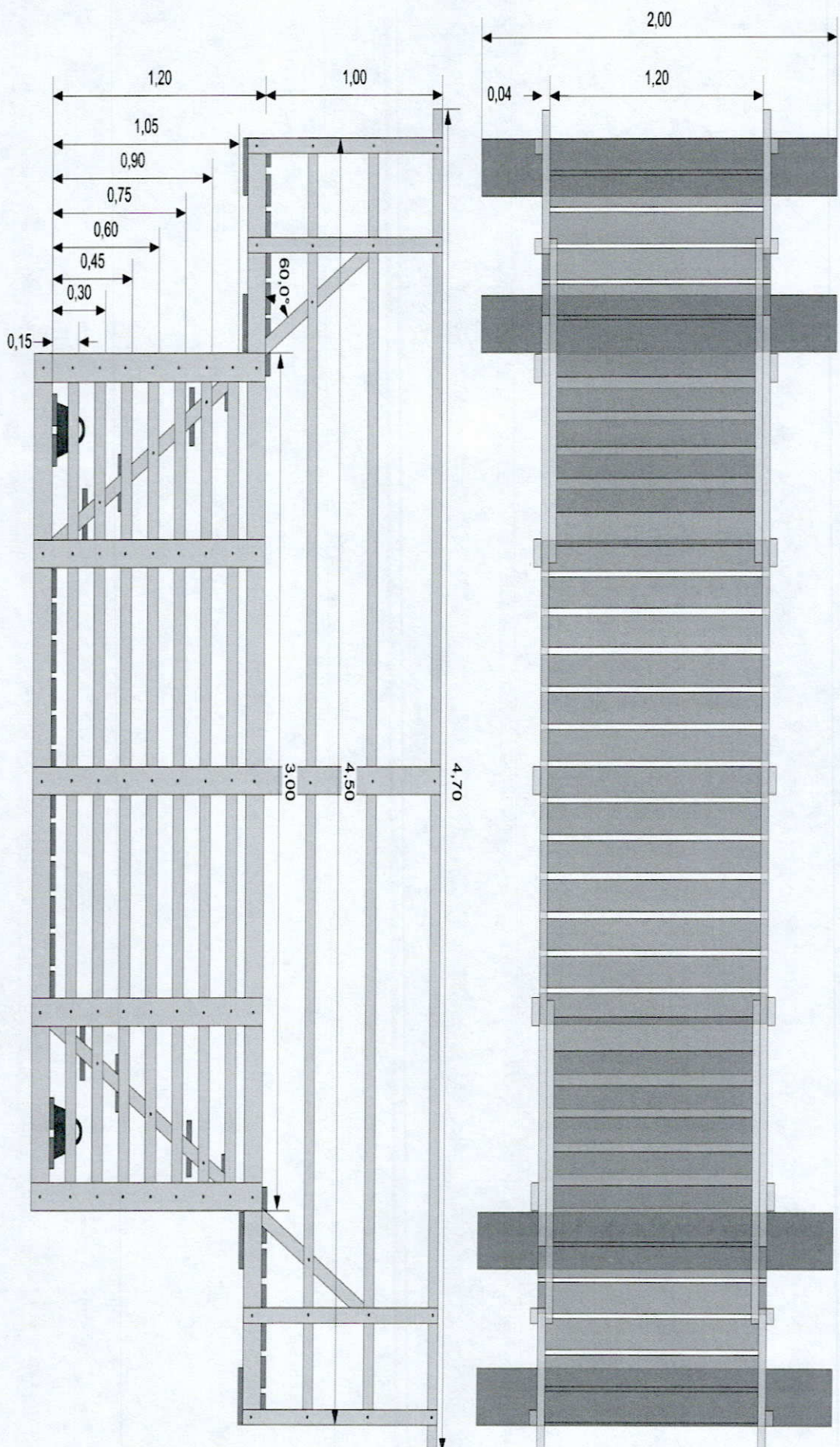
Чертеж конструкций мостков для Крещенских купаний на водных объектах (вариант 2)
